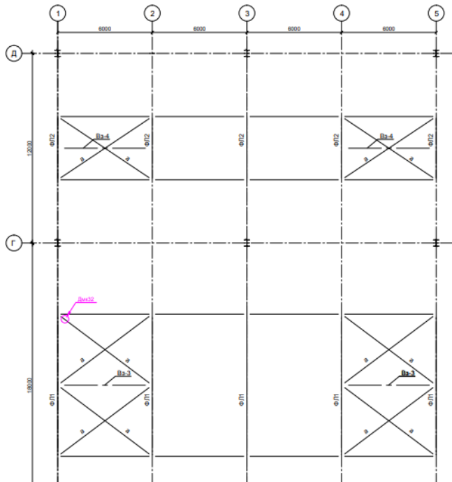
Схема розташування ферм ліхтарів, зв'язів по верхніх поясах ферм ліхтарів між осями 1-5 / В-Д
