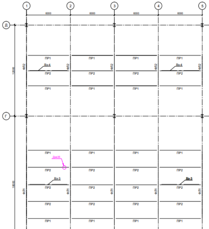
Схема розташування прогонів по верхніх поясах ферм ліхтарів між осями 1-5 / В-Д
