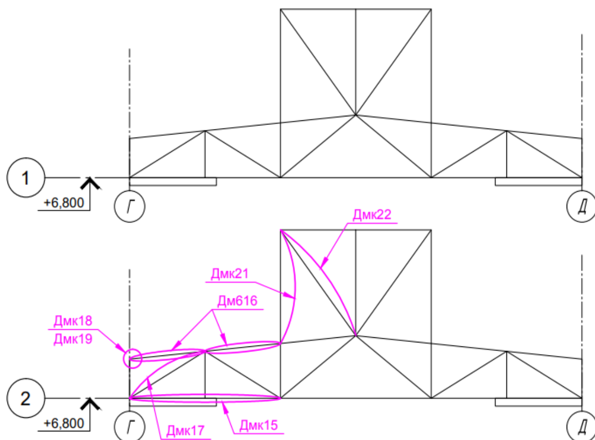
Схема розташування підкрівляних і кроквяних ферм, зв'язків по нижніх поясах ферм між осями 1-5 / В-Д
